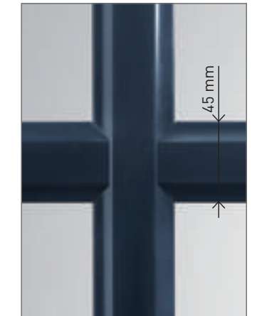
Petits bois ALU - Disponible en blanc, bicolore ou monocolore Section 45x8 mm
