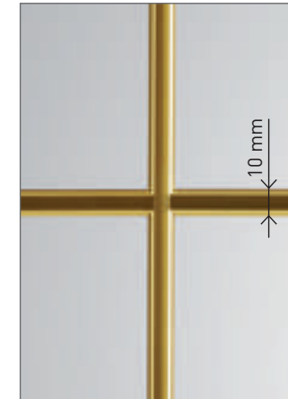
Petits bois LAITON TRADI Section 10x8 mm
